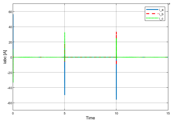
Figura 46: Corrientes i_{abc}(t)
