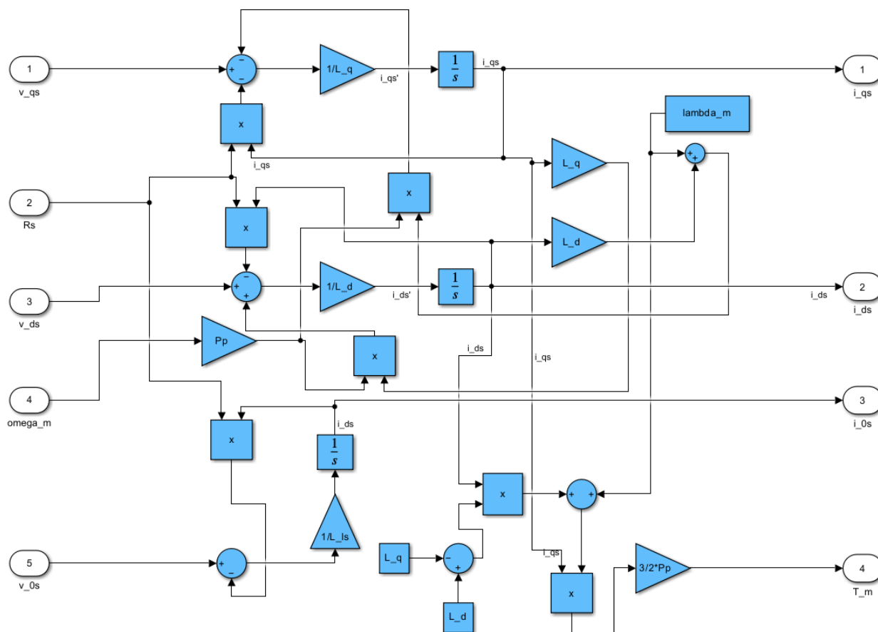
Figura 4: Subsistema electromagnético
